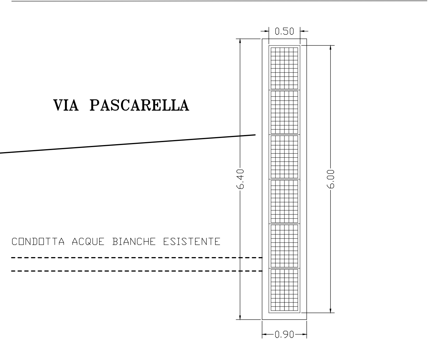
GRIGLIA TRASVERSALE ACQUE BIANCHE
